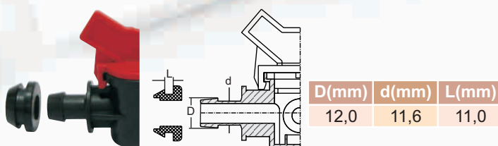
Grommet Γρόμμετ
