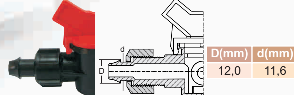
Offtake Πιπέτα
